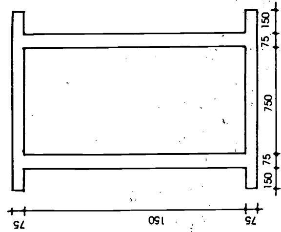
DOOR
