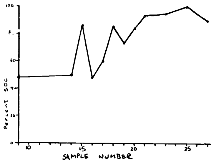
B. Uguisu: the SOC
