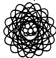
Uranium — 92 protons
