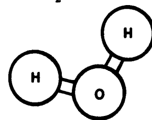
H_2O
