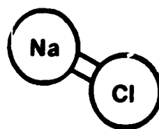
NaCl
