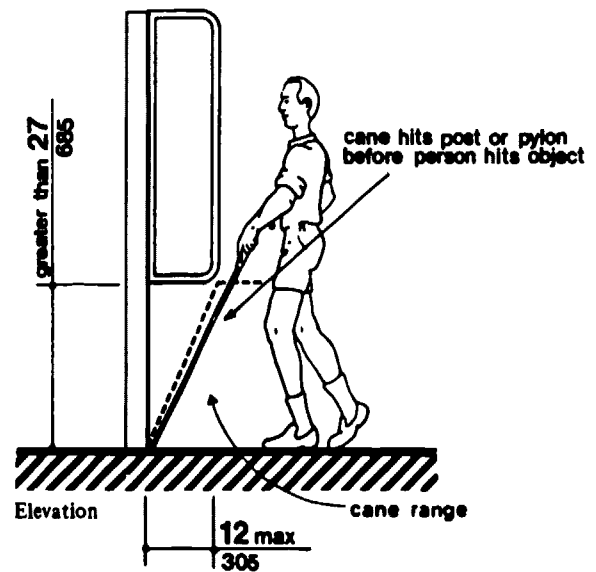
(d) Objects Mounted on Posts or Pylons
