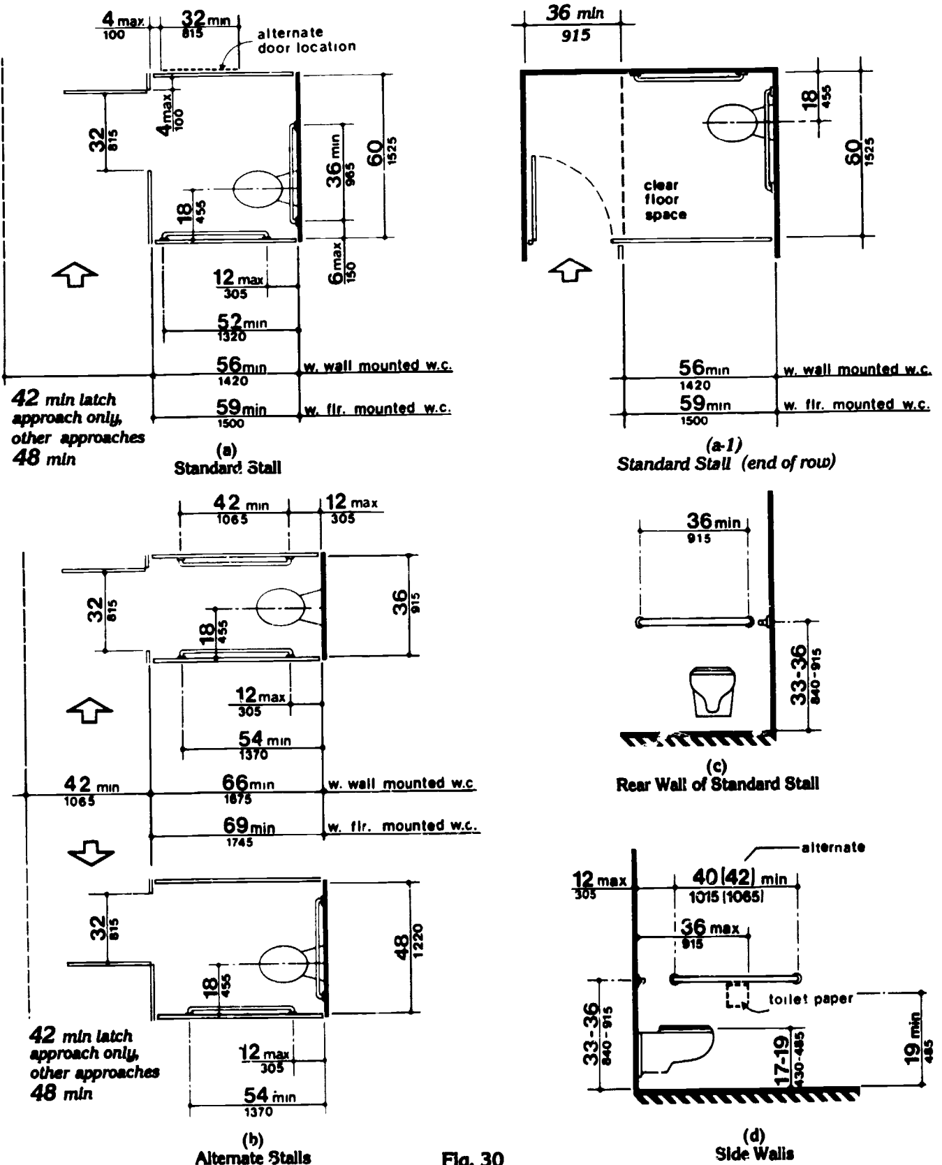
Fig. 30 Toilet Stalls
