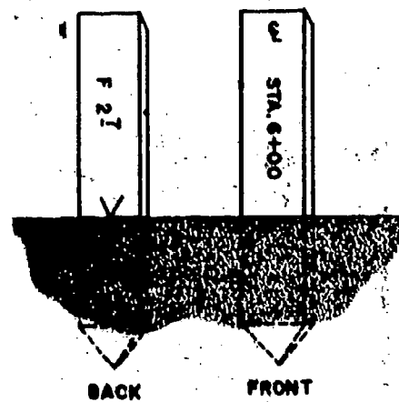
Fig 3-9. Fill stake.
