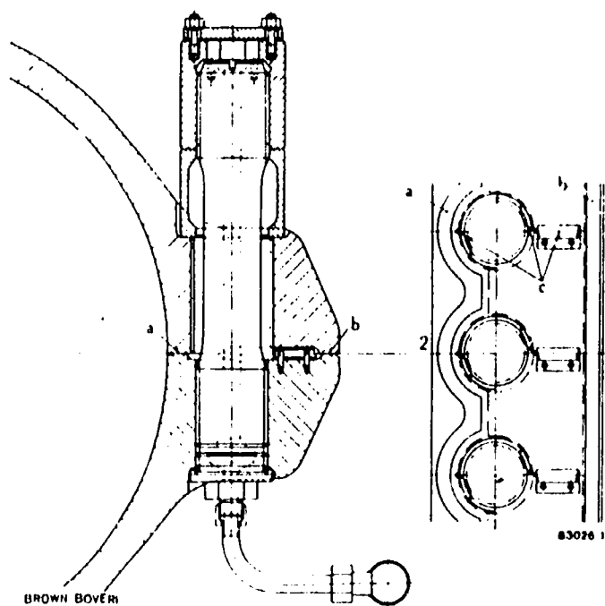
Fig. 18. — Flange warming
