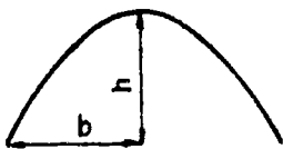
PARABOLA
