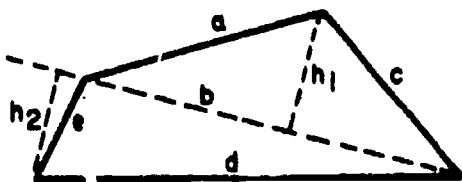
TRAPEZIUM
