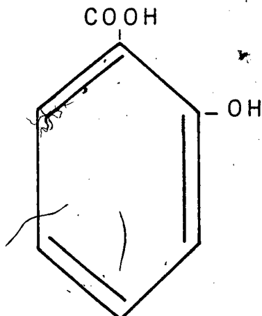
SALICYLIC ACID (ortho-hydroxybenzoic acid)
