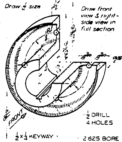
Flange
