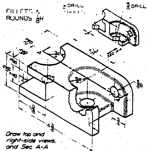
Pivot Base
