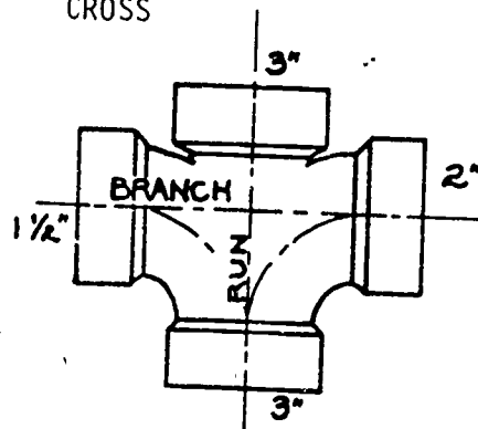
3X3X2X1½ CROSS
