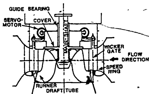
a. Francis-Type
