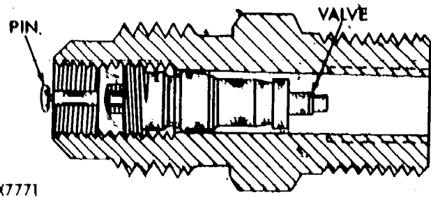
Fig. 42 — Schrader Valve
