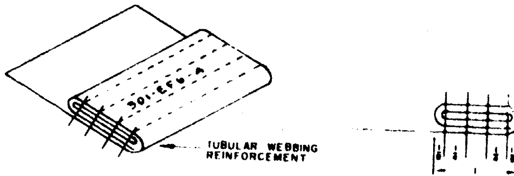
Figure 4. Edge Finishing Stitch, Efb-4.
