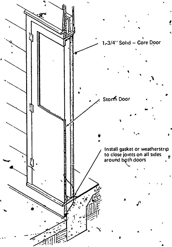
Fig. 5-4. DOOR MODIFICATIONS
