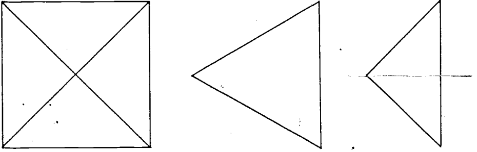
FIG. 36 (Model 1, p. 28)
