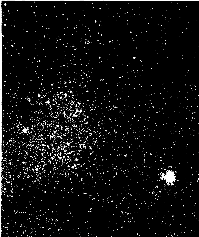
Figure 2-2 Gegenschein
