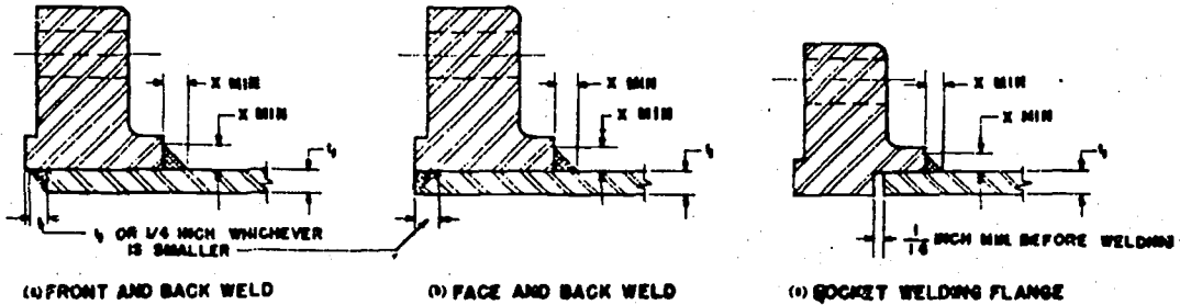
FIG 127.4.A FILLET WELD SIZE
