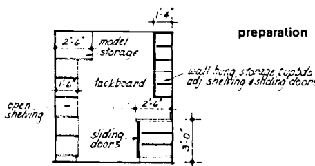
elevation L
