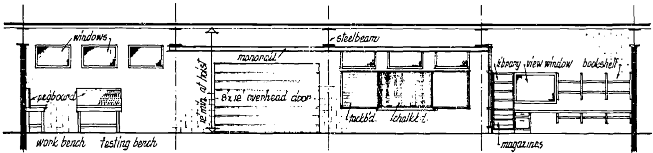
elevation A
