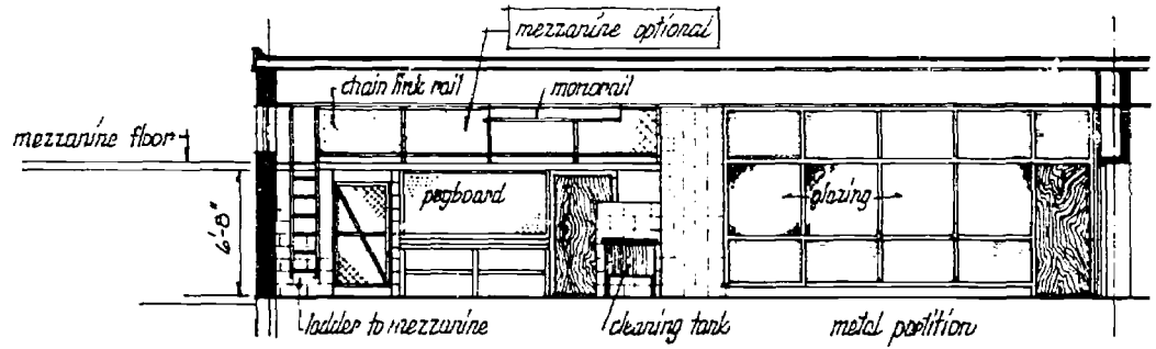
elevation B
