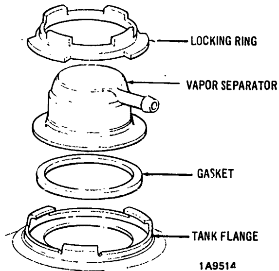
VAPOR SEPARATOR ASSEMBLY (EXC. TORINO & MONTEGO)
