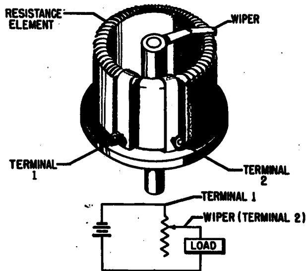
Figure 10-8.—Rheostat.
