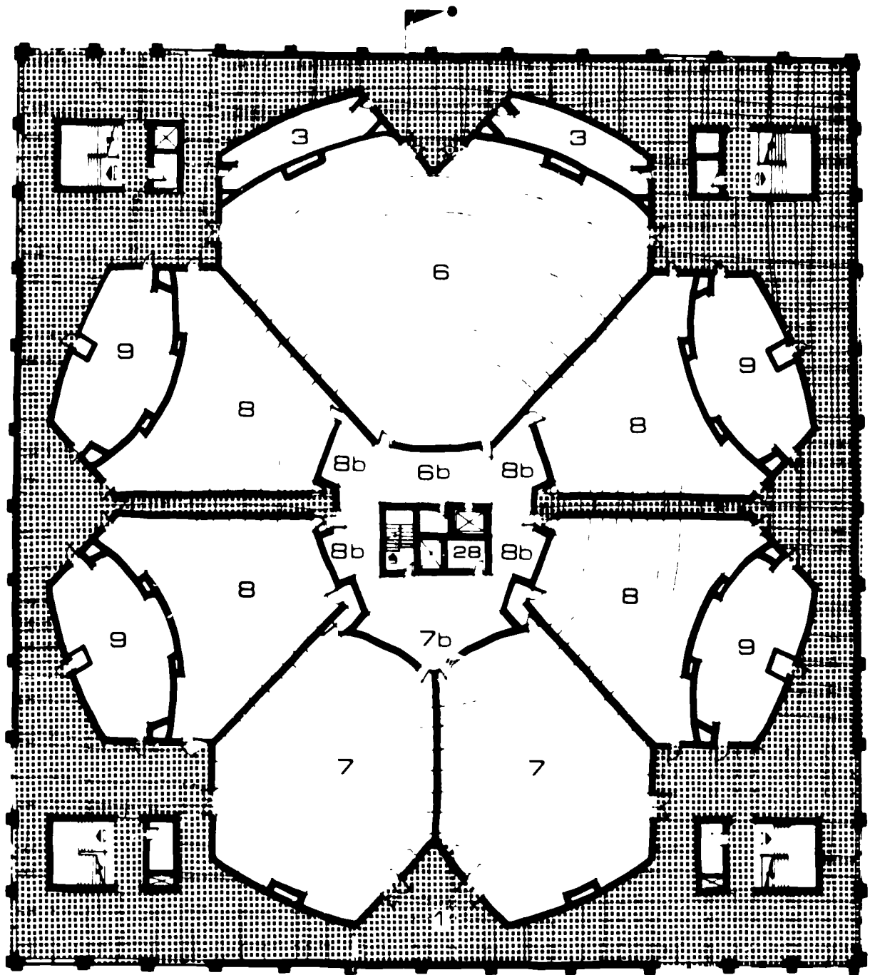
COMMONS LEVEL PLAN
