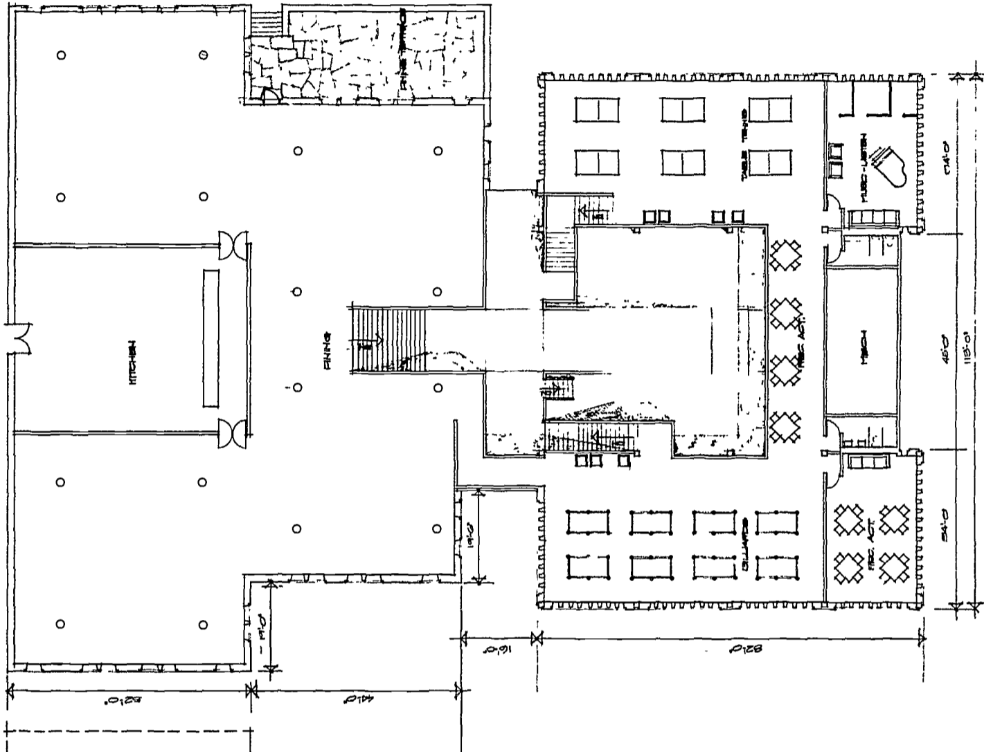
SECOND FLOOR PLAN COMMONS BLOCK 10
